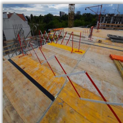
Barierki harmonijkowe wyznaczające strefy Szczepanowskiego R4R
