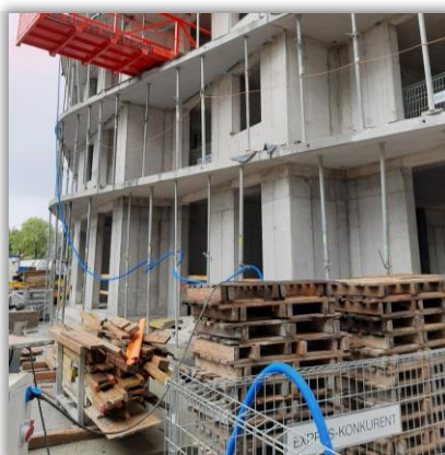
Linki zabezpieczające metalowe podpory KRK I
