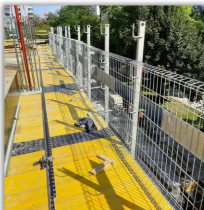
Prefabrykowane podesty szalunkowe MidPoint 71
